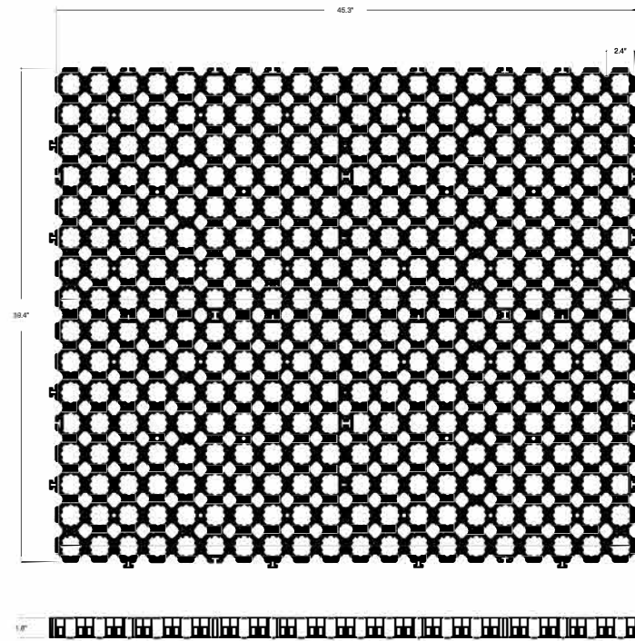
GD Gravel™ 60-40 : Surface Paving Grid Scale : N.T.S.
