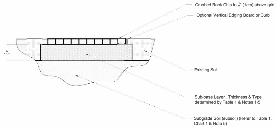
GD Gravel™ 60-40 : Surface Paving Grid Scale : N.T.S.
